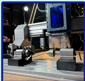
نصب روتاری
