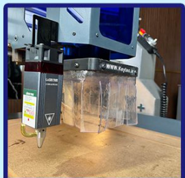
نصب ماژول لیزر
