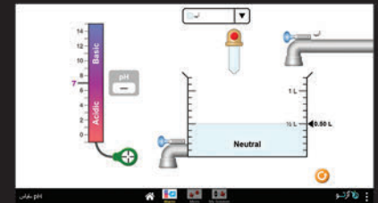
شبیه‌ساز سنجش PH
