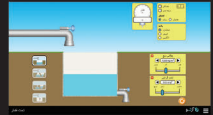
شبیه‌ساز فشار مایعات
