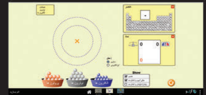
شبیه‌ساز ساخت اتم
