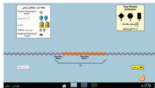
شبهه ساز بیان ژن
