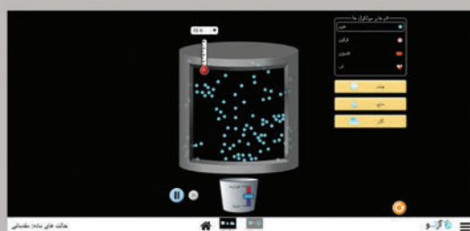
شبهه ساز حالت های ماده
